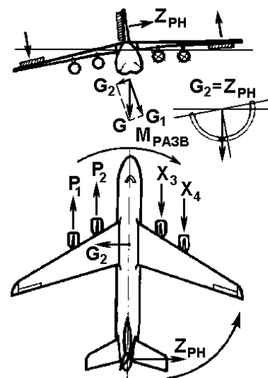
Рис. 19. Полет с креном
