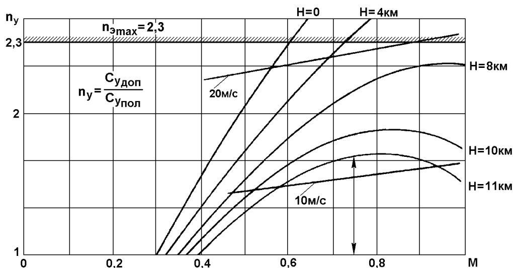
Рис. 38. Максимально допустимые перегрузки в зависимости от числа М
