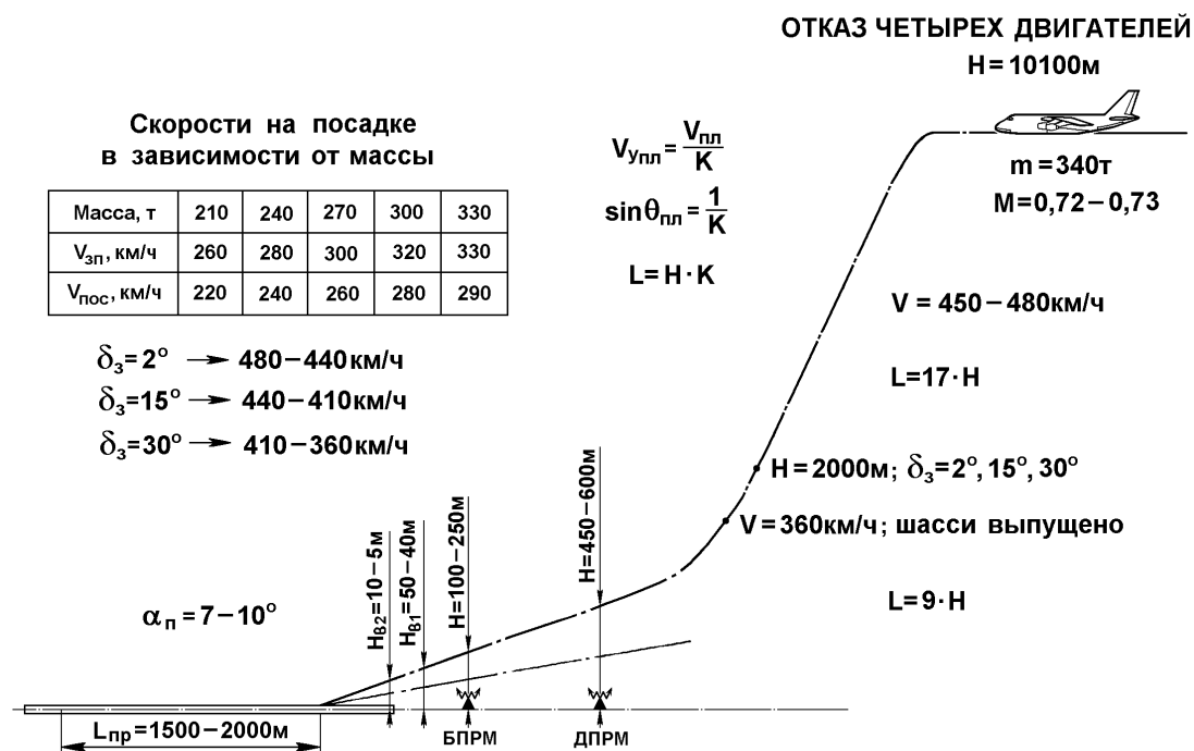
Рис. 35. Полет ВС с четырьмя отказавшими двигателями
