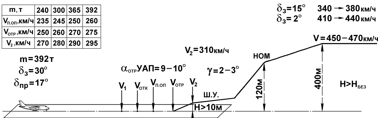
Рис. 23. Продолженный взлет ВС
