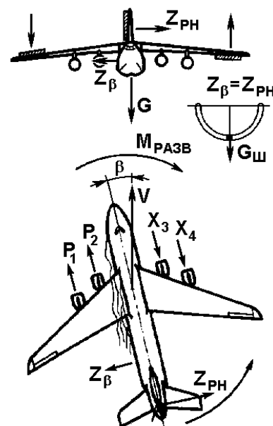
Рис. 20. Полет со скольжением
