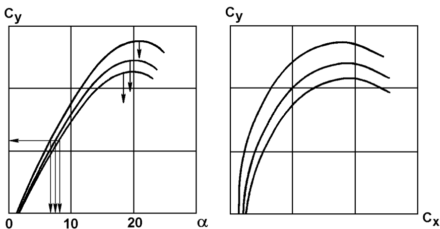
Рис. 41. Влияние обледенения на полярю ВС
