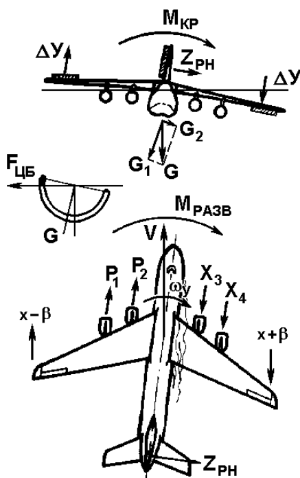
Рис. 18. Поведение ВС при отказе двигателя
